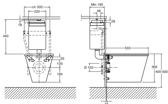
Ifö mini inbyggnadscistern
