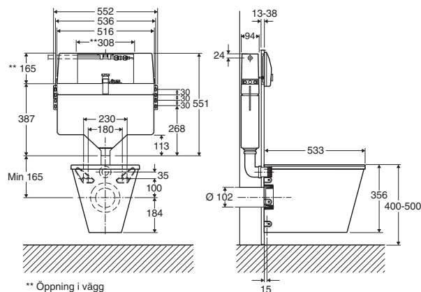
Ifö Premont cistern, standardmodell
