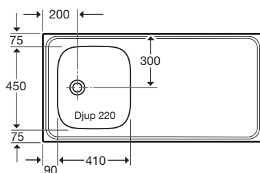
Ifö Compact Allbänk CABM 12 RM. Blandare från FMM.
