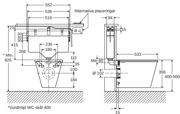
Ifö Premont cistern, låg modell
