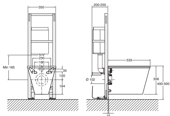
Ifö WC-element 1100 MC4 med mini cistern
